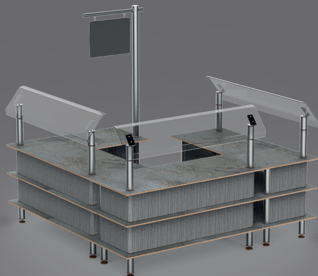
CLASSIC STATION SELF SERVICE MIT SCHILD, HAUCHSCHUTZ UND COVERS STATION CLASSIC SELF-SERVICE AVEC PANCARTE, PARE-HALEINE ET HOUSSES L 255 CM B 255 CM H 239,5 CM
